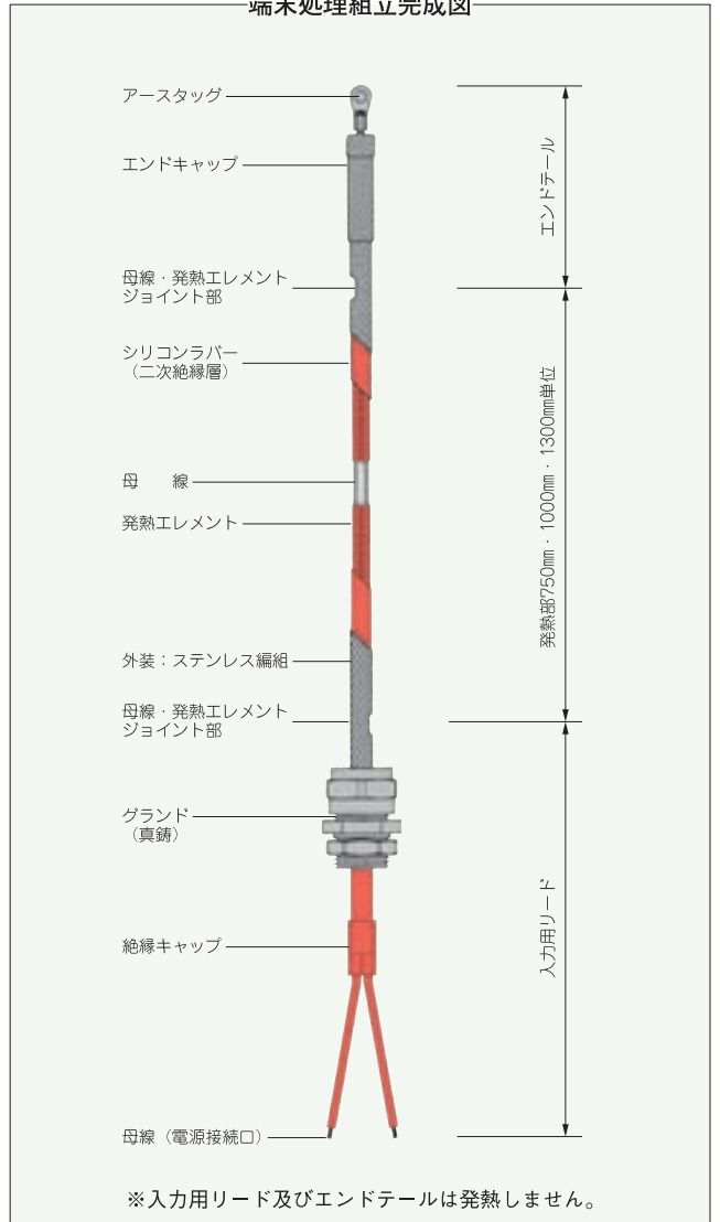
端末処理組立完成図
