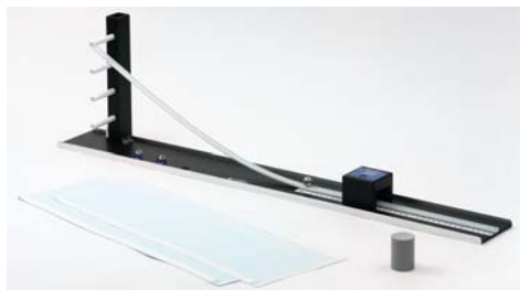
54034 衝突実験器セット CF-BV(2個組)
